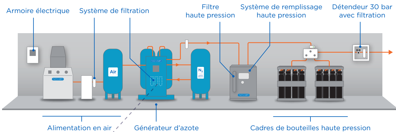
Exemple de chaîne de production d'azote pour la découpe laser
